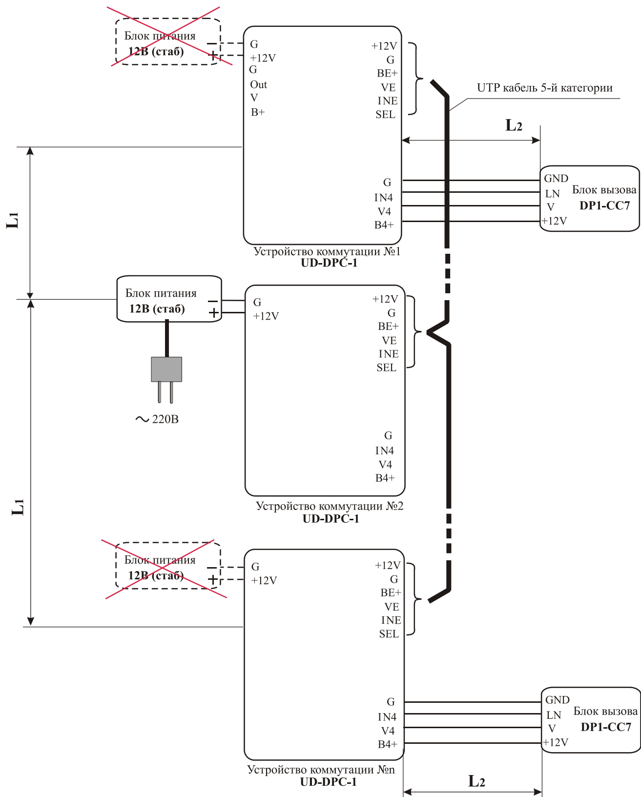
Рис.4 Пример подключения БП в группе УК.
