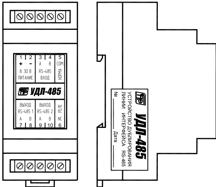
Рис.1. Внешний вид устройства и расположение клемм
