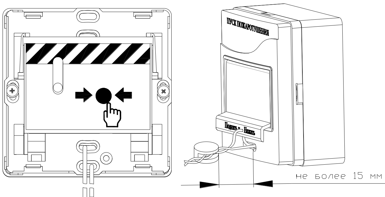
Рисунок 2.2.3.2 Пломбировка УДП
