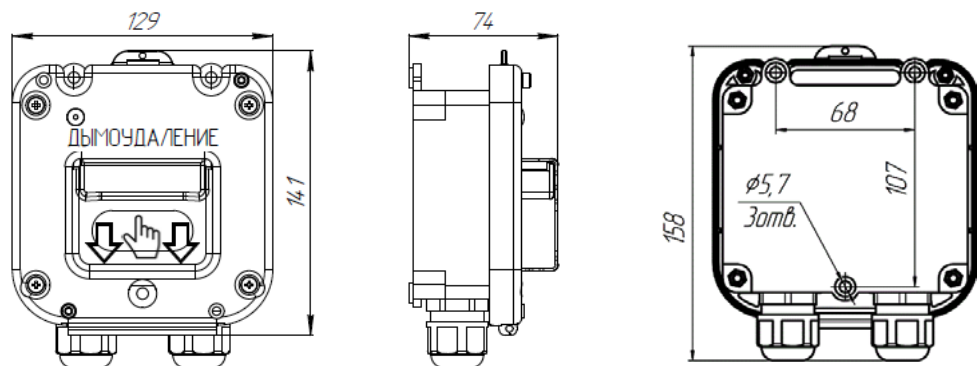
Рис.3. Габаритные размеры устройства
