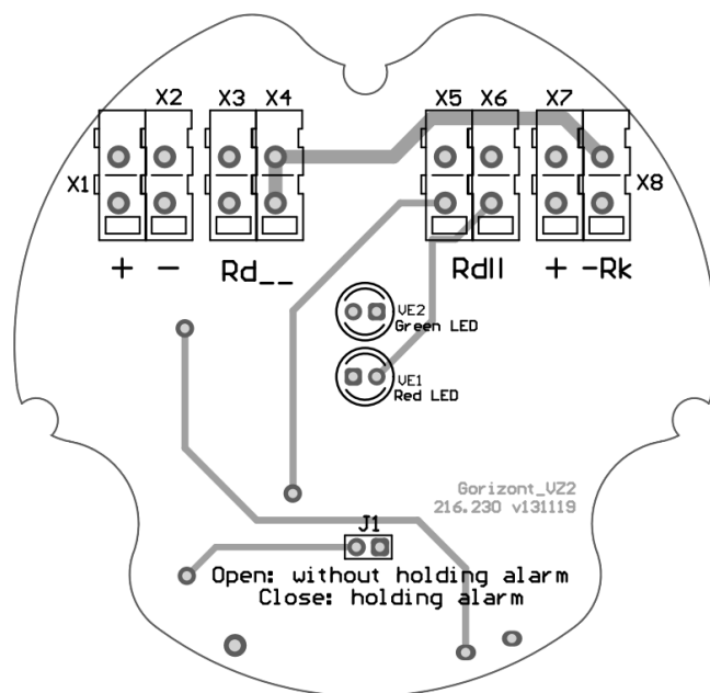
Рис.А4 Внешний вид платы извещателя
