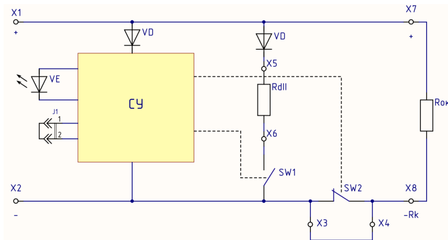
а) параллельное включение извещателей
