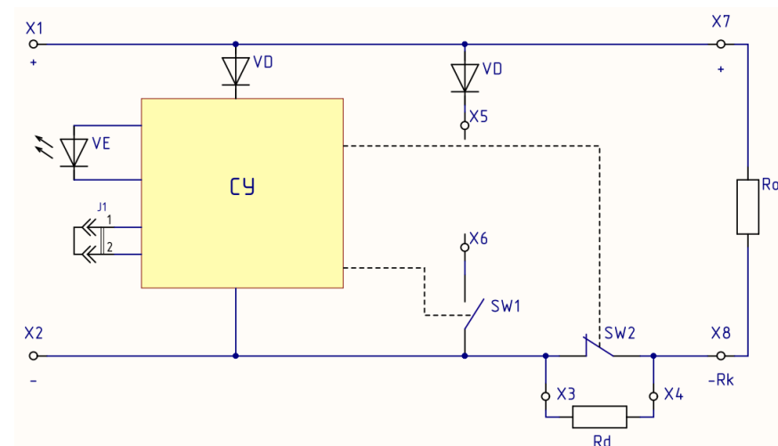
Рис.А3 Принципиальная электрическая схема извещателя
