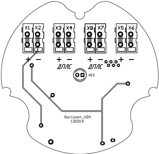
Рис.А7 Внешний вид платы адресного извещателя
