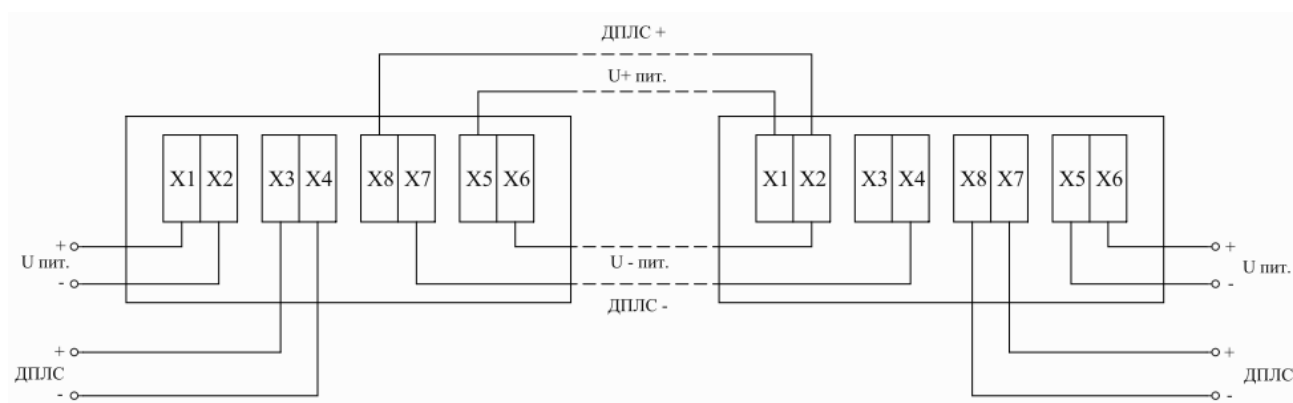
Рис.А8 Схема подключения адресных извещателей ИПР 535 Халзан-Ех (УДП 535 Халзан-Ех)
