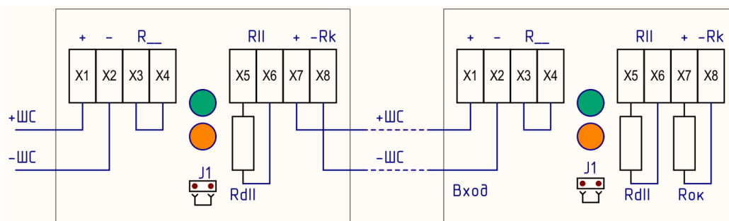
а) параллельное включение извещателей
