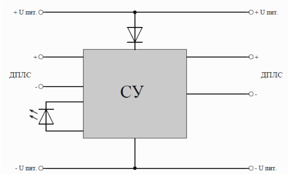
Рис.А6 Принципиальная электрическая схема адресных извещателей
