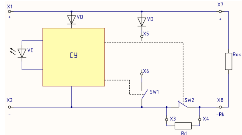
б) последовательное включение извещателей
