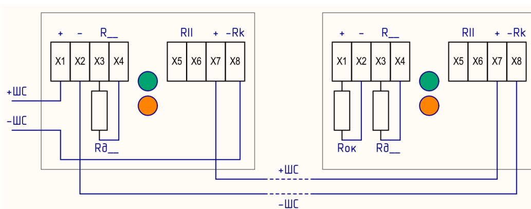
в) последовательное включение, знакопеременное напряжение ШС
