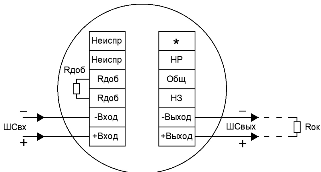
Рисунок 5 – 2-х проводная схема подключения с использованием режима неисправность
