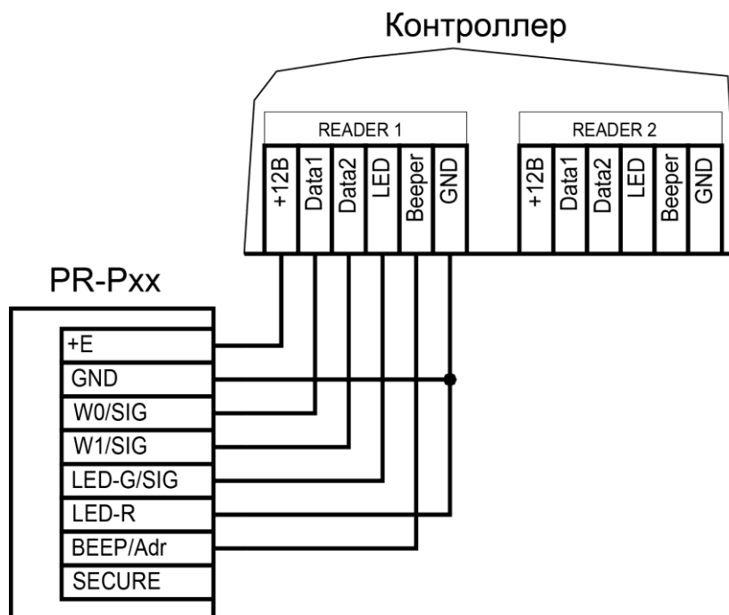
Рисунок 4. Подключение считывателя в режиме Wiegand 26
