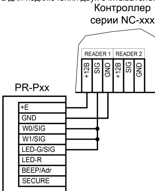
Рисунок 5. Подключение считывателя в режиме Parsec, адрес 1 (внутренний)
