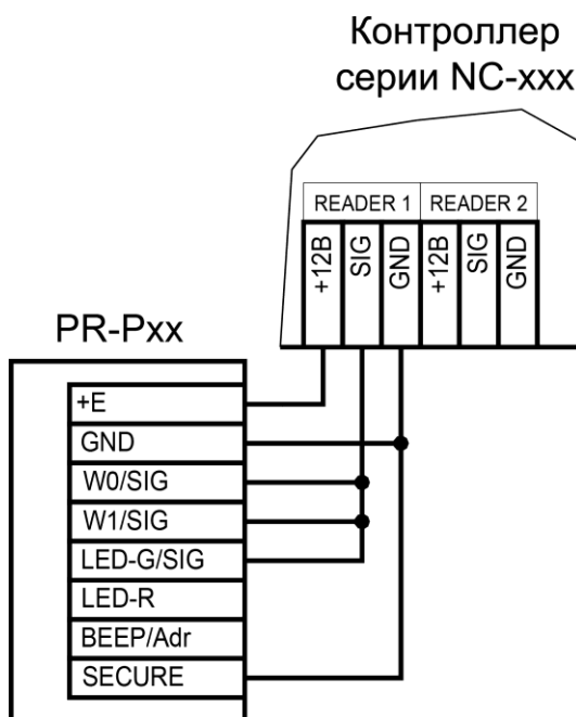
Рисунок 7. Включение защищенного режима на примере считывателя, подключенного в режиме Parsec с адресом 1
