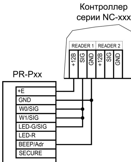
Рисунок 6. Подключение считывателя в режиме Parsec, адрес 0 (наружный)
