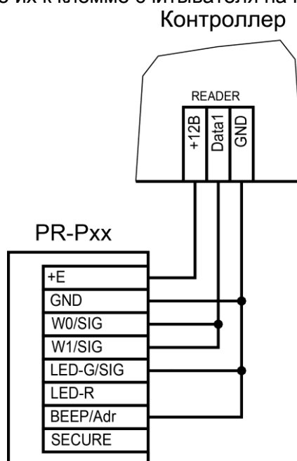
Рисунок 3. Пример подключения считывателя в режиме Touch Memory
