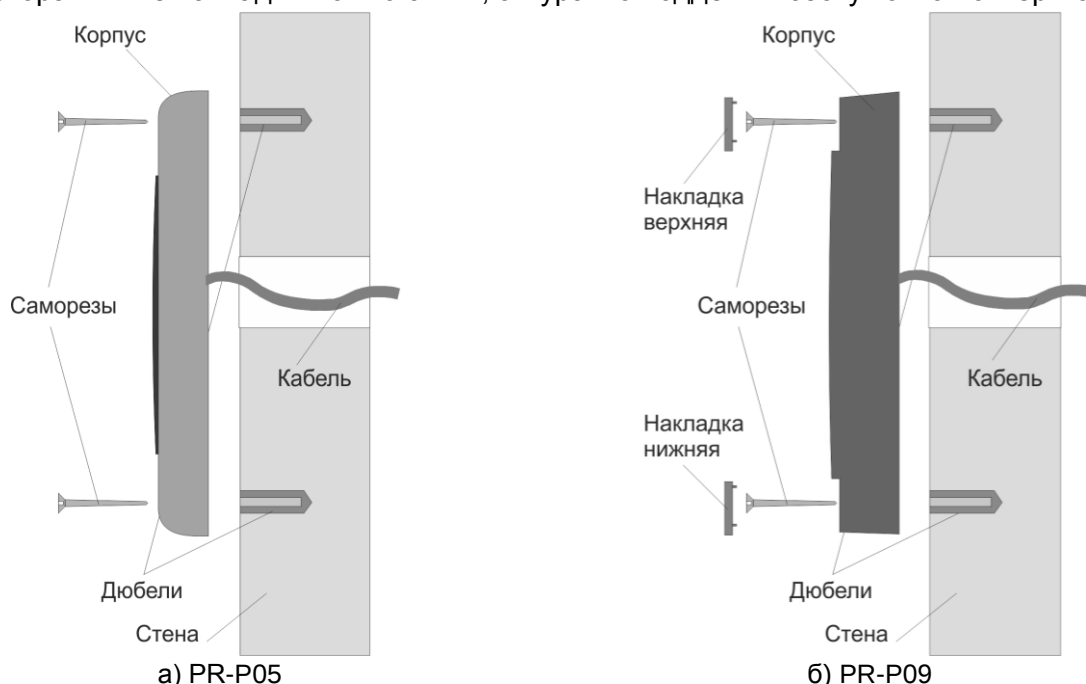
Рисунок 2. Крепление считывателей
