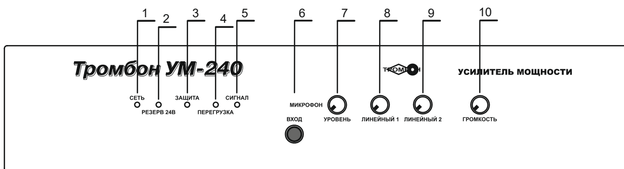
Рисунок 1 – Внешний вид передней панели Усилителя
