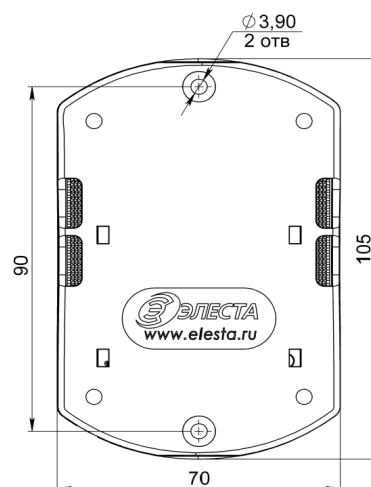
Рисунок 2. Габаритные и установочные размеры прибора
