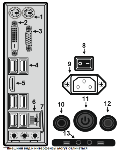
Рисунок 2. Назначение элементов системного блока.
