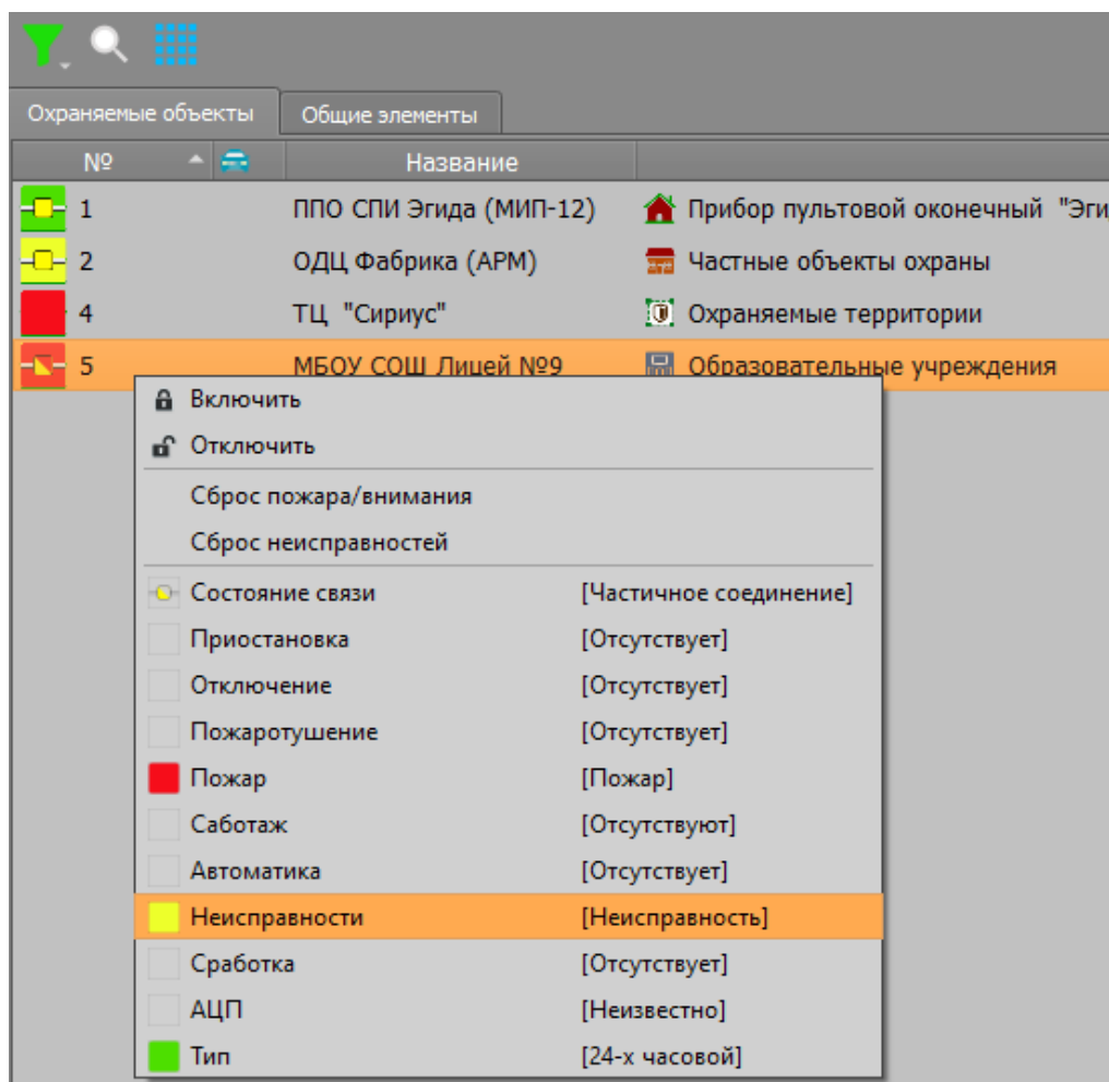
Рисунок 197 Пример отображения мультисостояния адресного извещателя С2000-КДЛ
