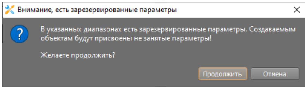
Рисунок 48 Окно предупреждения
