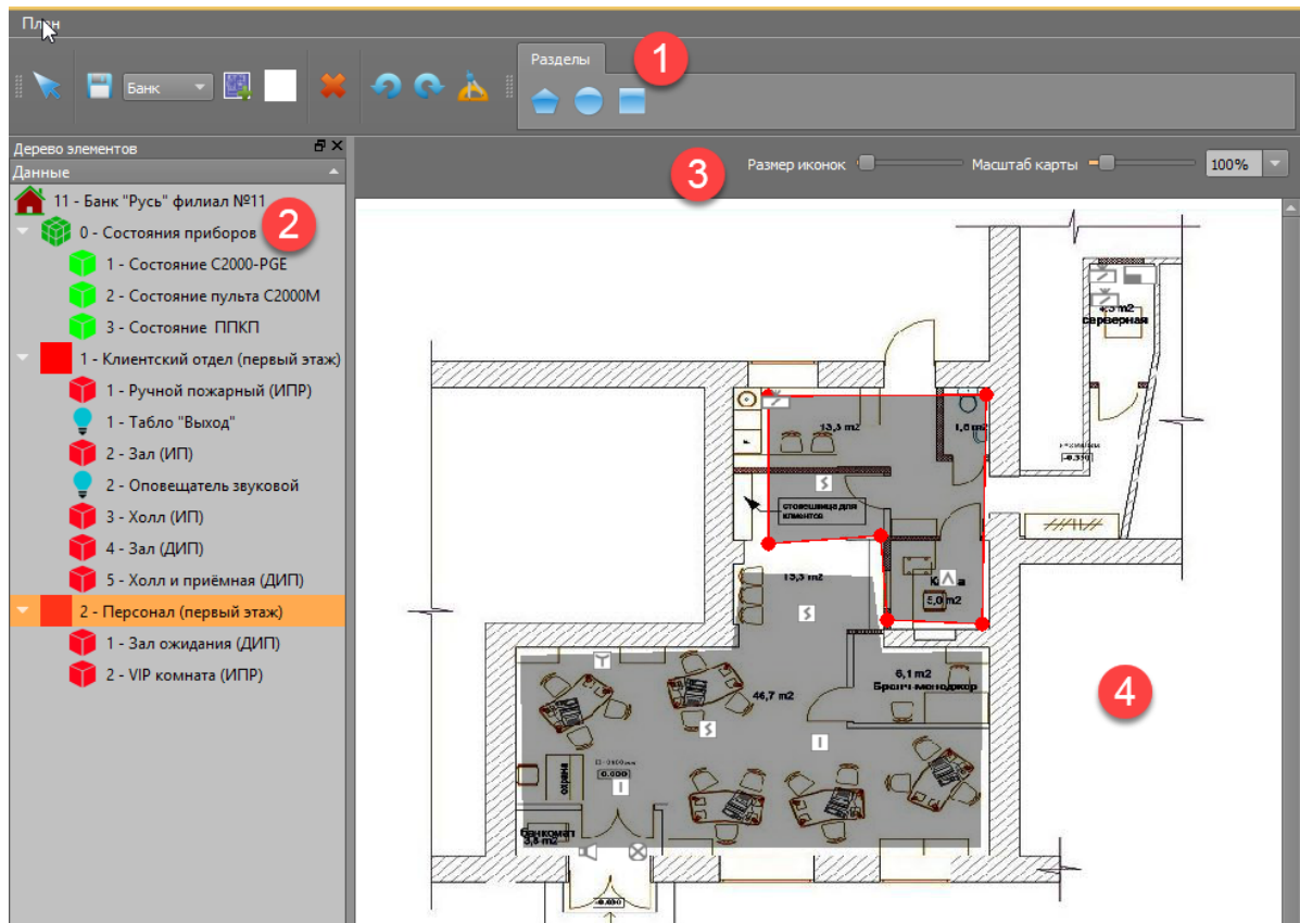
Рисунок 128 Окно редактора планов
