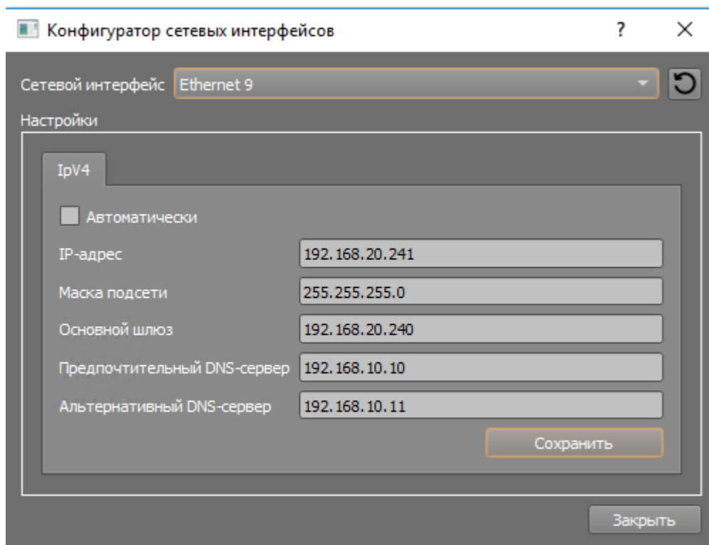
Рисунок 24 Конфигуратор сетевых интерфейсов ППО КСПИ Эгида
