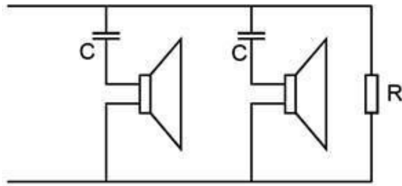
Рис. 4.5. Подключение речевого оповещателя в системе EVA
