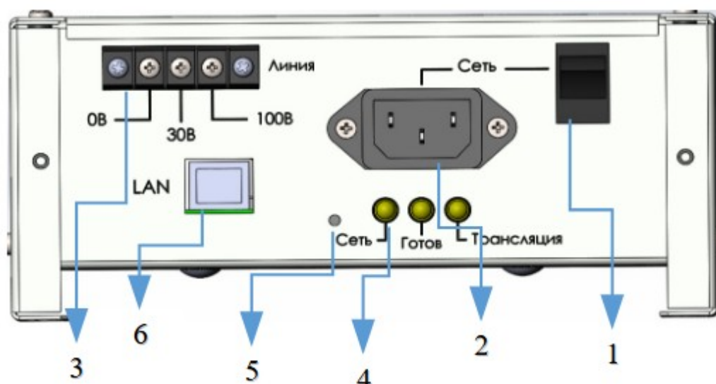
Рисунок 2 - Коммутационный отсек, вид снизу
