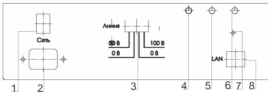
Рисунок 2 - Коммутационный отсек
