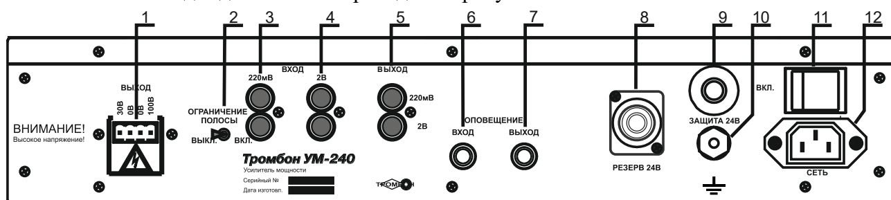
Рисунок 2 – Внешний вид задней панели Усилителя
