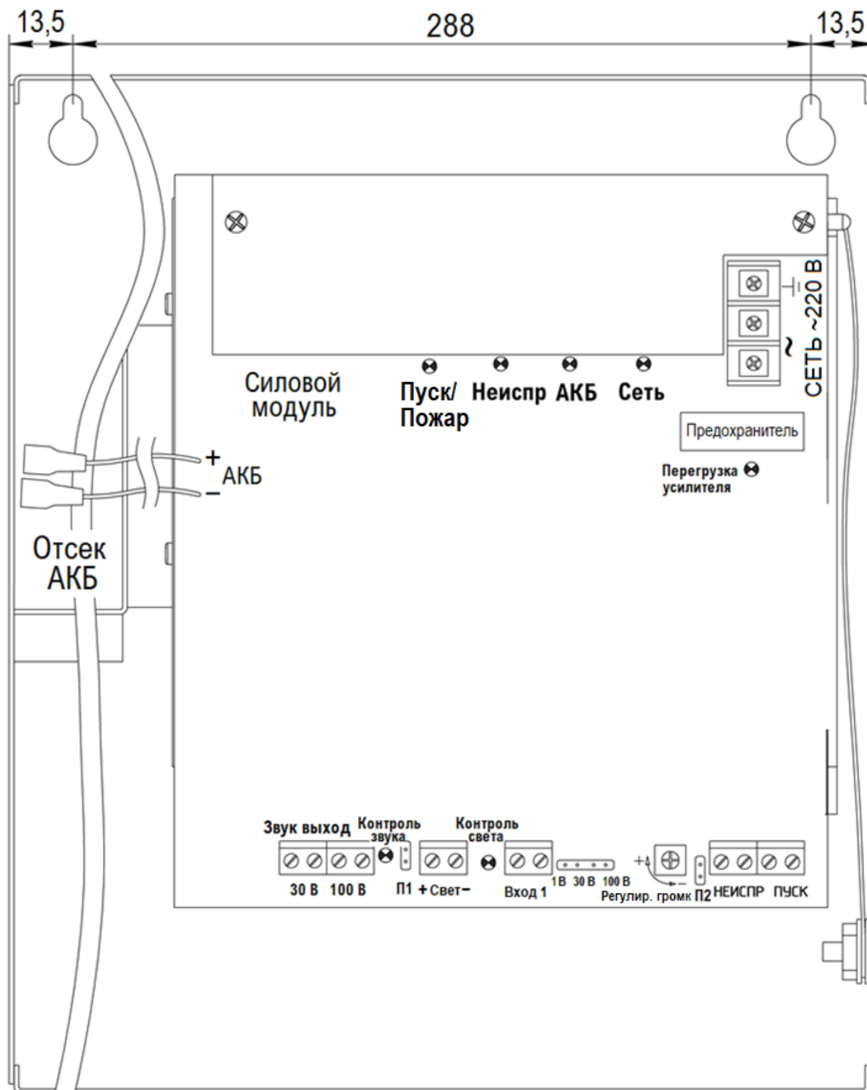
Рисунок 1 - Общий вид линейного усилителя «Октава-100Б» со снятой крышкой
