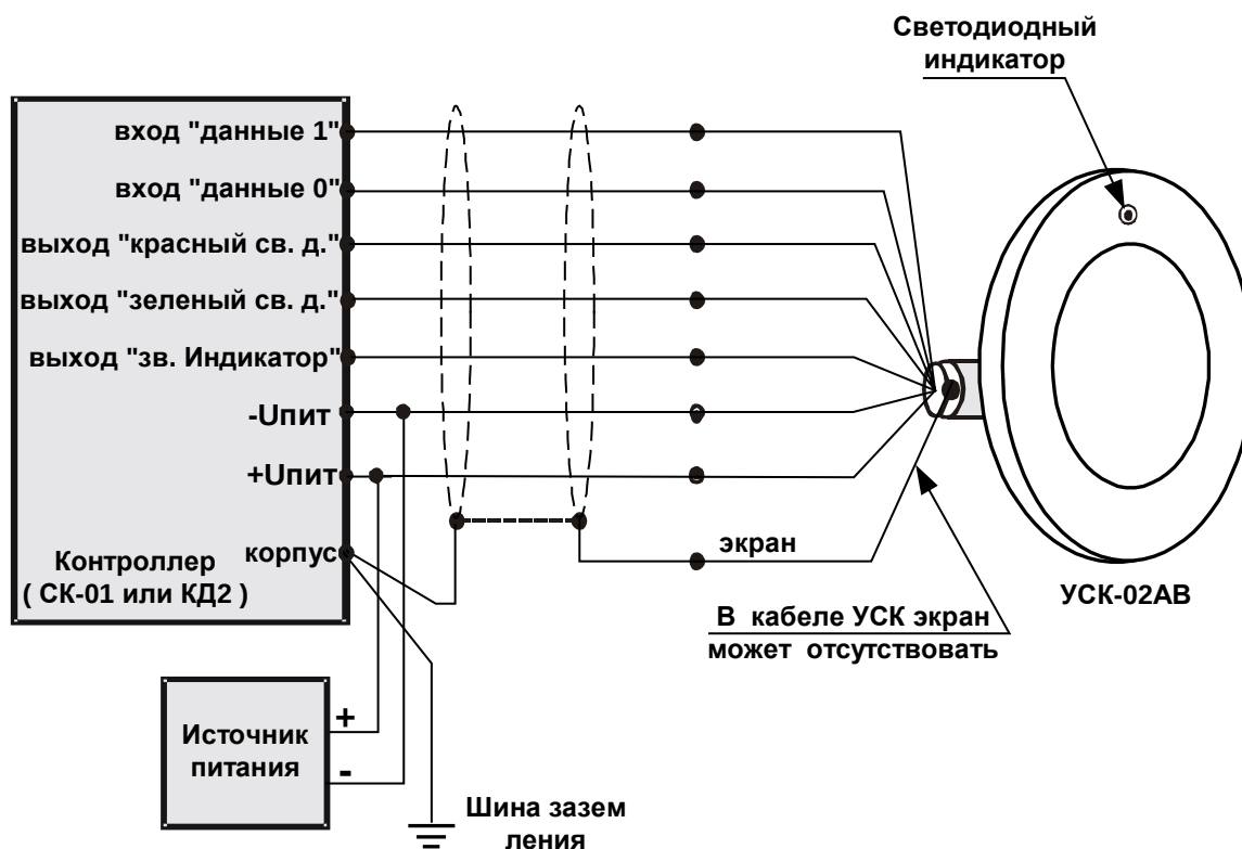
Рис. 2 Схема подключения УСК-02АВ
