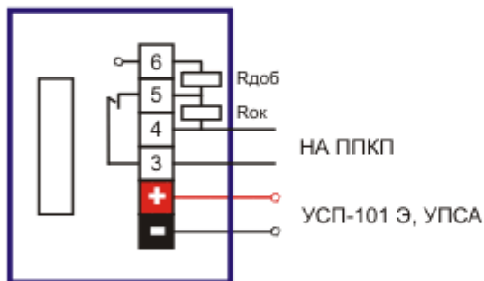
Схемы подключения УСП-101 через релейный блок.
