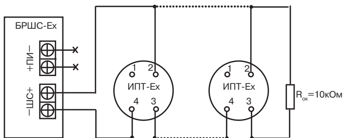
Рисунок 51 — Рекомендуемая схема подключения ИПТ-Ех к БРШС-Ех (в один шлейф БРШС-Ех рекомендуеся включать не более 10 ИПТ-Ех)
