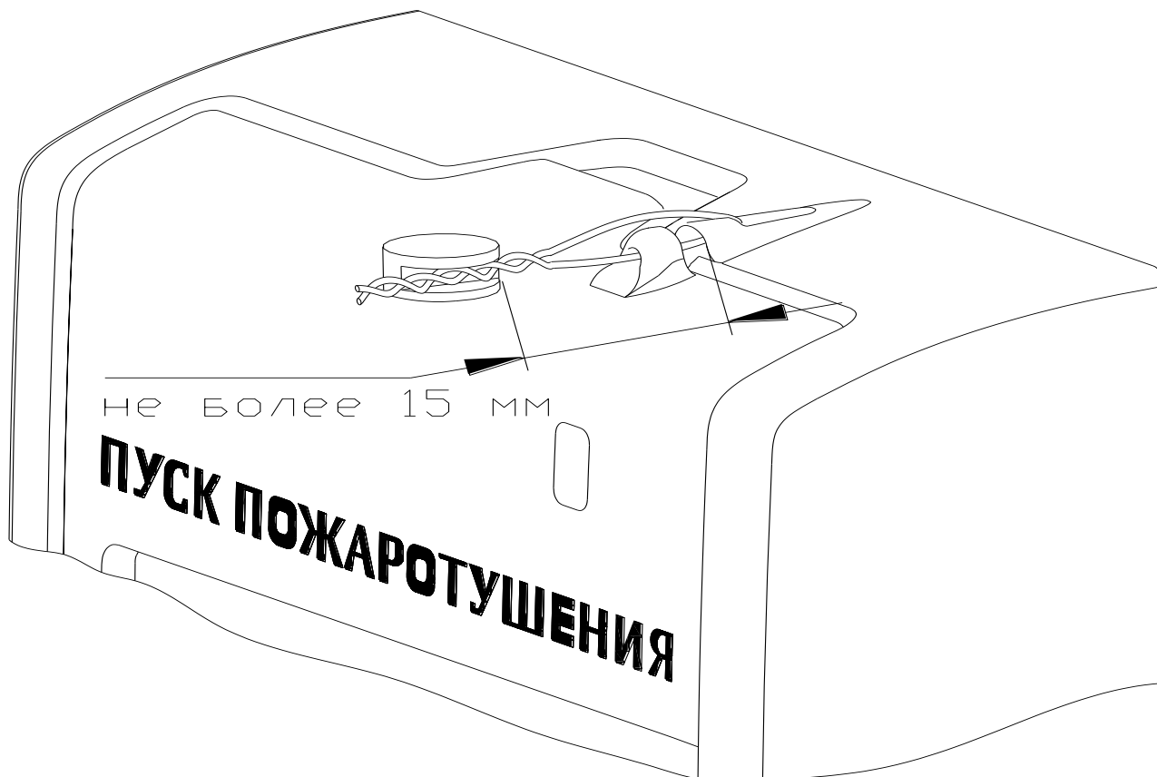
Рисунок 2.2.3.2 Пломбировка УДП
