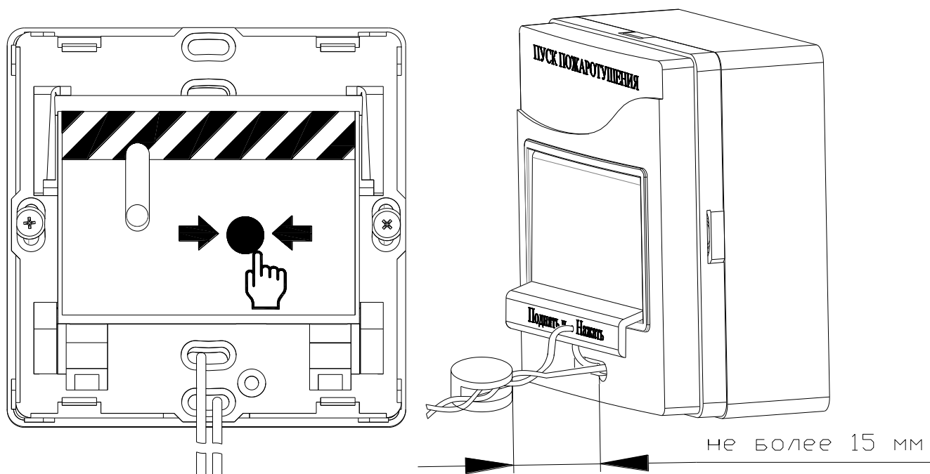
Рисунок 2.2.3.2 Пломбировка УДП
