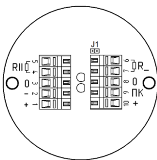
Рисунок 4. Внешний вид платы ИП535-07е-“ПУСК”-И2.
