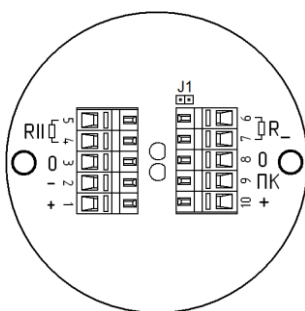
Рисунок 4. Внешний вид платы ИП535-07с-“ПУСК”-И2-О.
