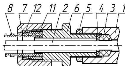
монтаж кабелем в металлорукаве KB15, KB18, KB20
