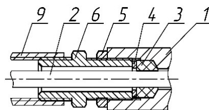
Рисунок 4 – Кабельный ввод
