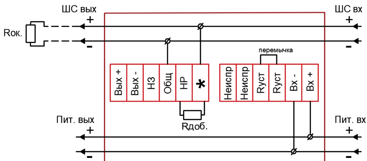
Рисунок БЗ – 4-х проводная схема подключения без контроля НЕИСПРАВНОСТИ.
