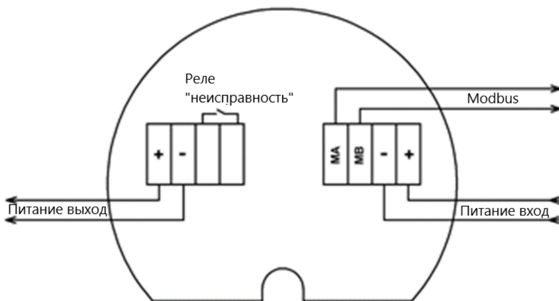
Рисунок Б1 – Схема подключения по протоколу Modbus
