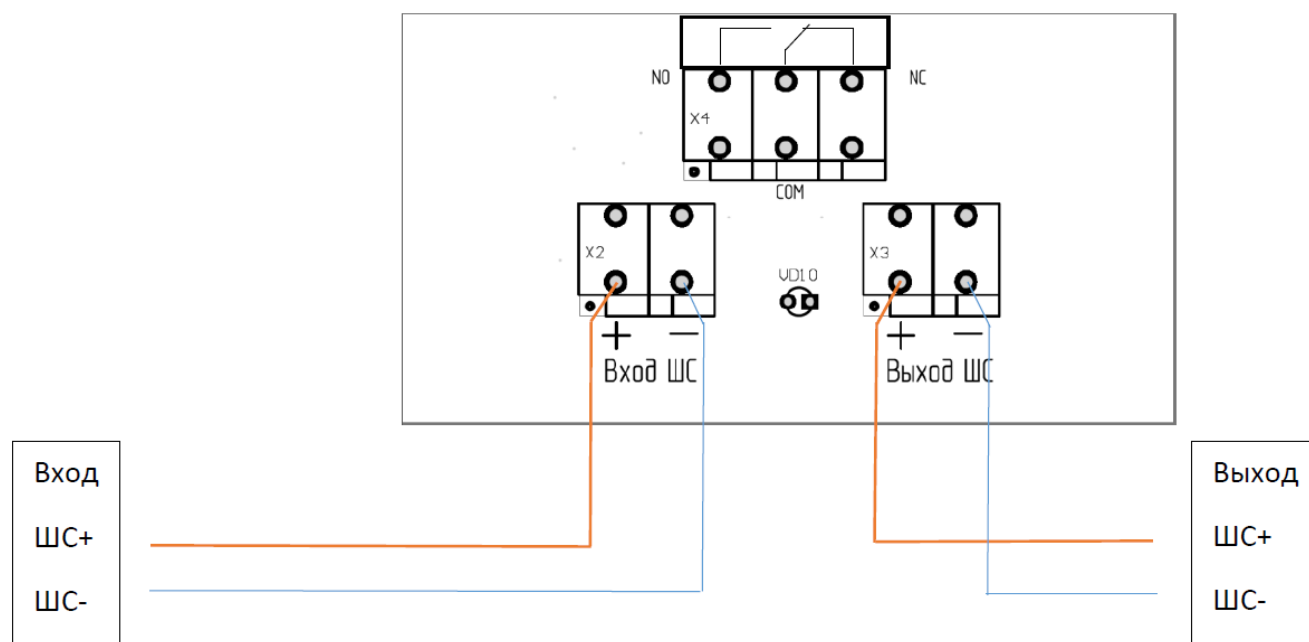
Рисунок Б2 – схема подключения «Спектрон-513-Ехi-М-УДП-03»
