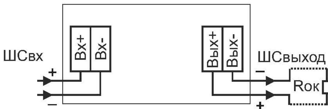
Рисунок Б1 – схема подключения «Спектрон-513-Ехi-М-УДП-01», «Спектрон-513-Ехi-М-УДП-02»
