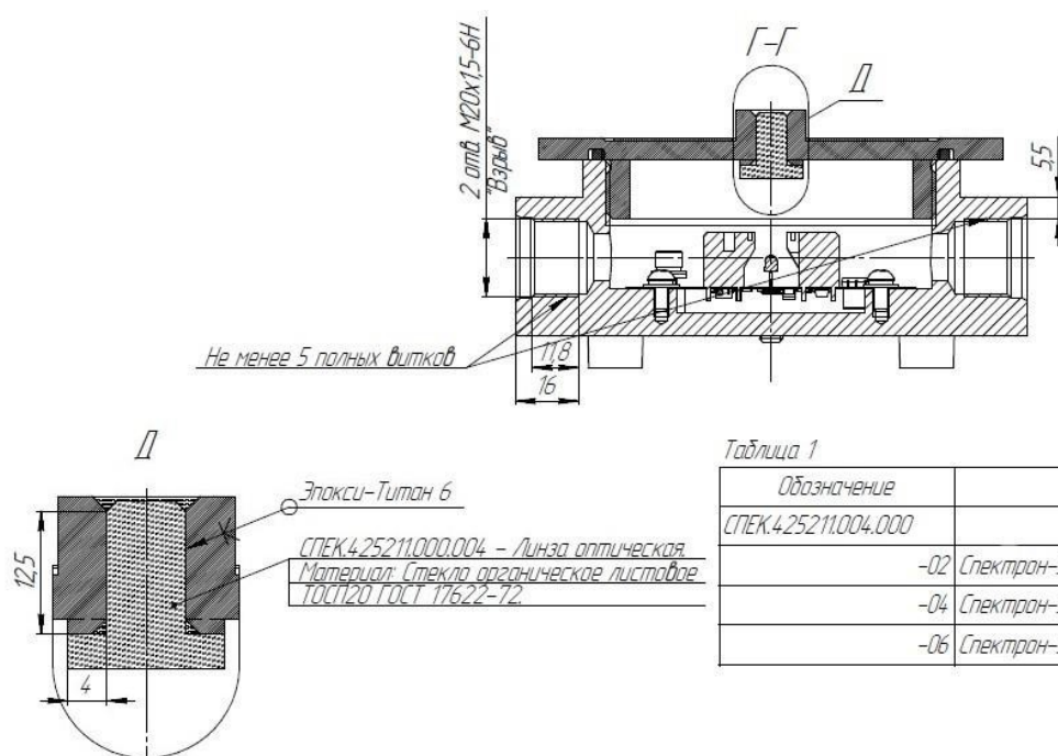
Рисунок А3 – Чертеж безопасности «Спектран-535-Exd-H-УДП-01/02/03»
