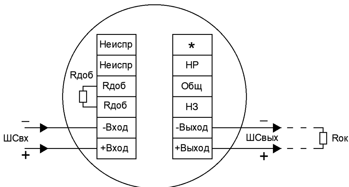
Рисунок Б2 – 2-х проводная схема подключения с использованием режима «НЕИСПРАВНОСТЬ»
