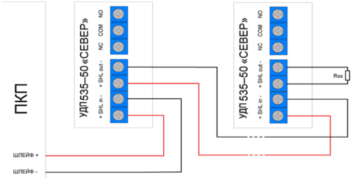
Рис.2. Схема подключения устройств в шлейф
