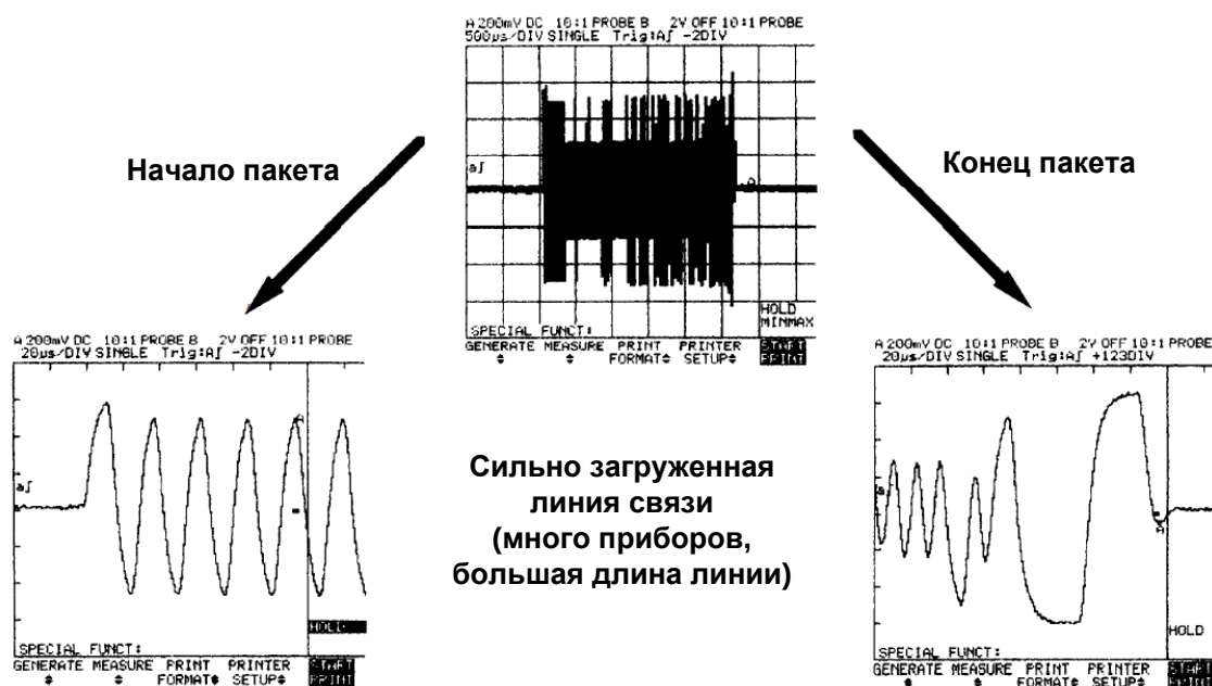
Рисунок 60 Типичная осциллограмма сигнала при большой нагрузке линии связи
