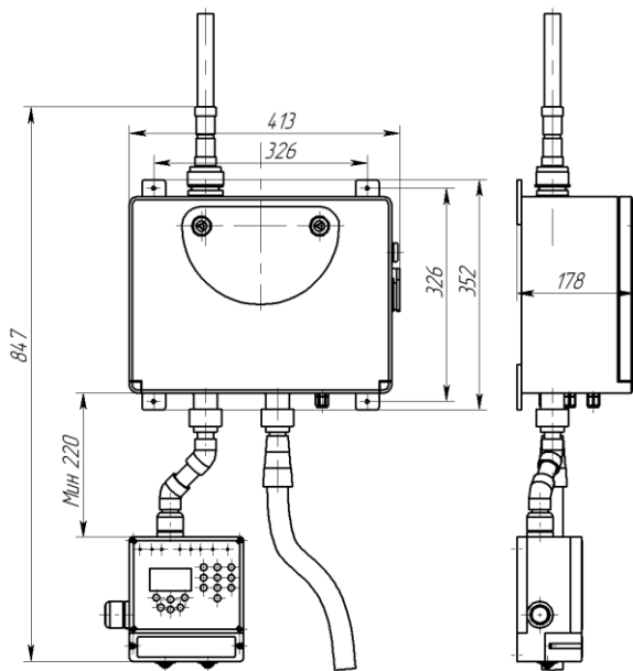
Рисунок 4 – Габаритные и монтажные размеры
