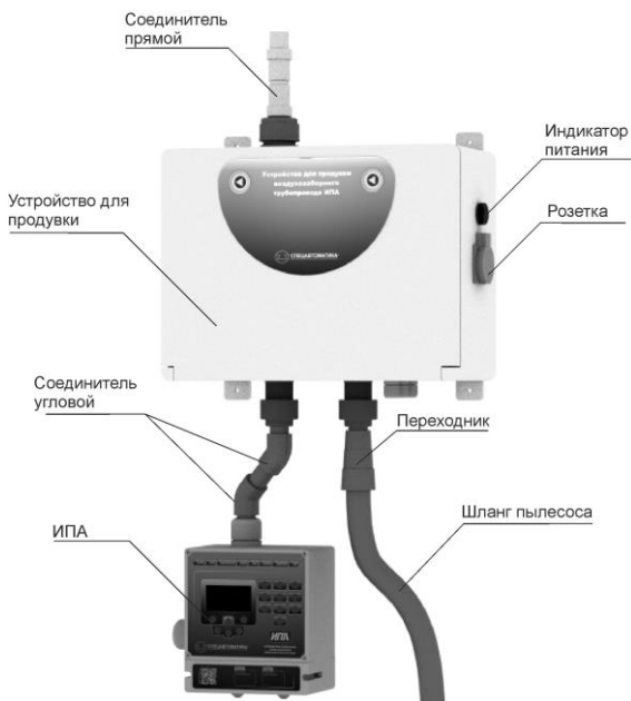
Рисунок 2 – Устройство, подключенное в аспирационную систему
