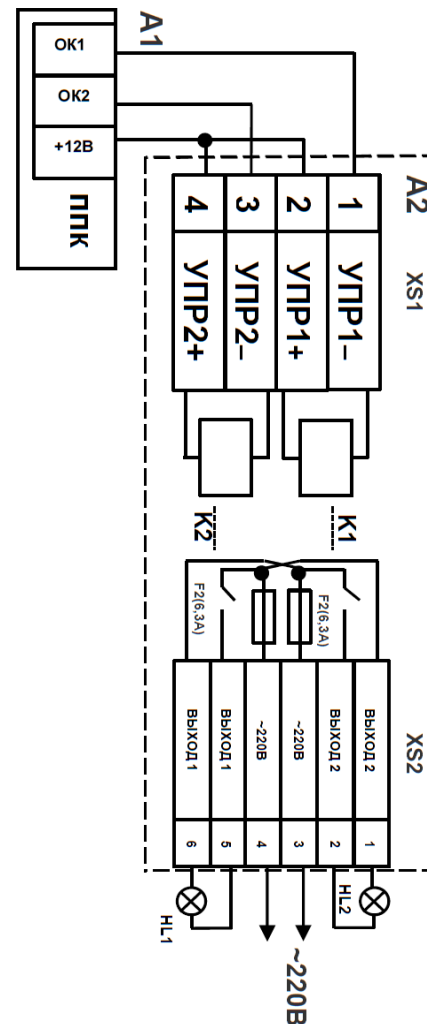
Рисунок 1 - Схема подключения для исполнений УК-20 и УК-20/1 к выходу ППК с открытым коллектором (ОК)
