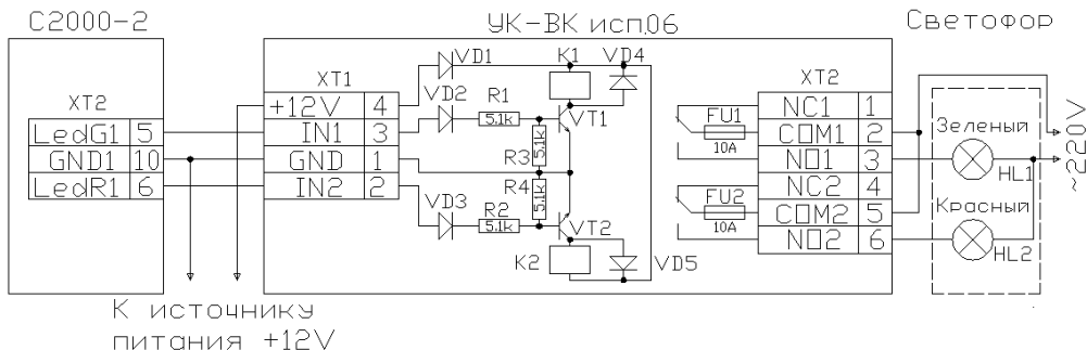
Рисунок 1 Схема подключения «УК-ВК исп.06» к контроллеру «С2000-2» для управления светофором в режиме «Шлагбаум»
