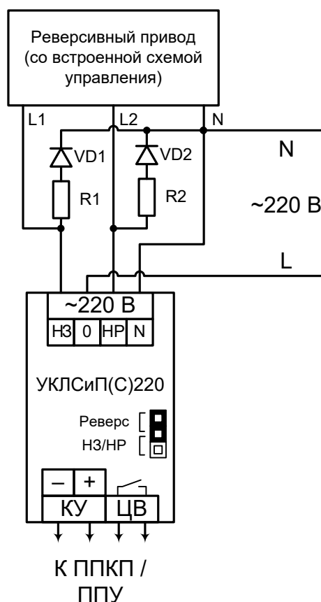
Рисунок 5 Примеры схем подключения реверсивных исполнительных устройств к УКЛСиП(С)220
