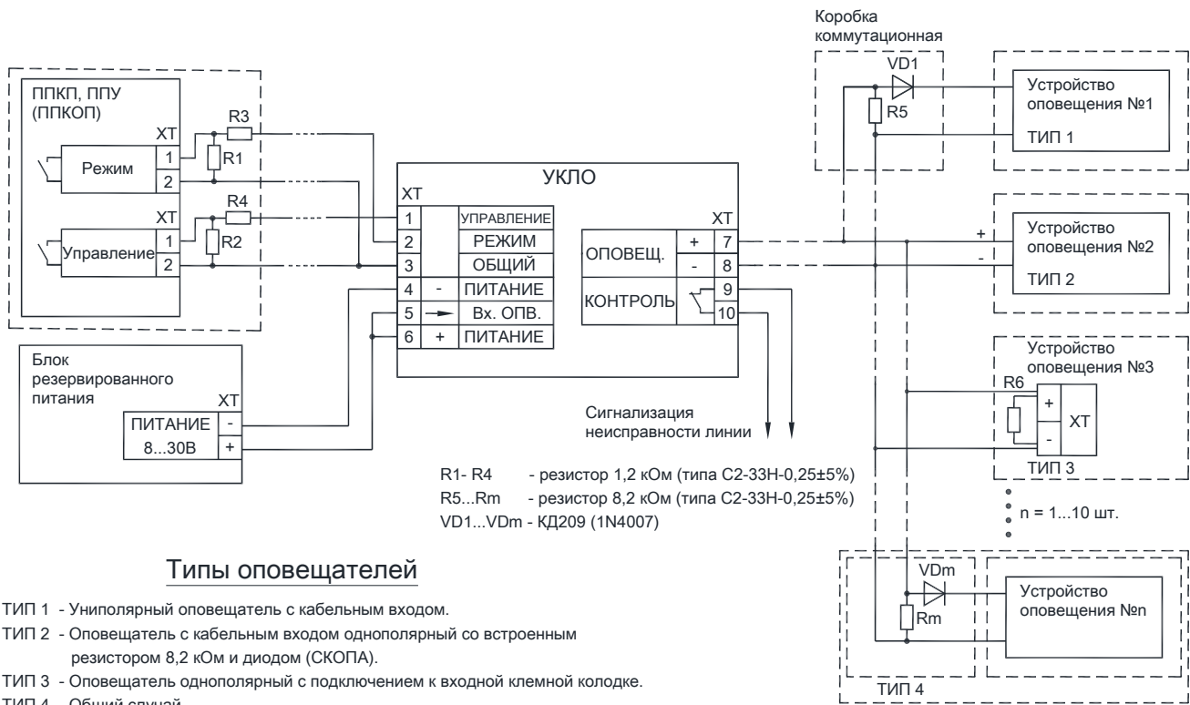
Рис. 2. Схема подключения УКЛО. (Схема подключения нескольких УКЛО к одному ПУ представлена на сайте www.specpribor.ru )
