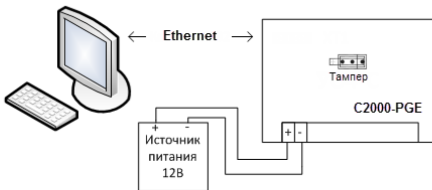
Рисунок 2. Подключение «C2000-PGE» к сетевой плате ПК через кабель Ethernet
