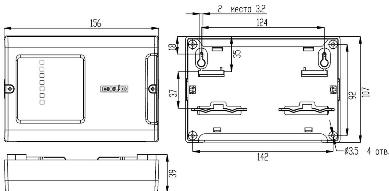
Рисунок 8-1 Габаритные размеры
