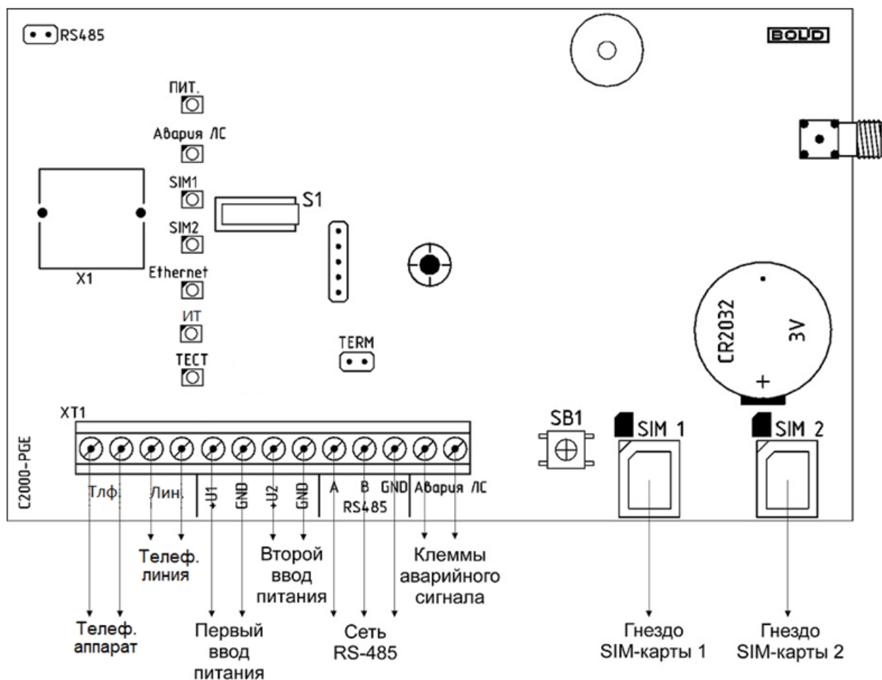
Рисунок 8-4 Схема подключений «C2000-PGE»
