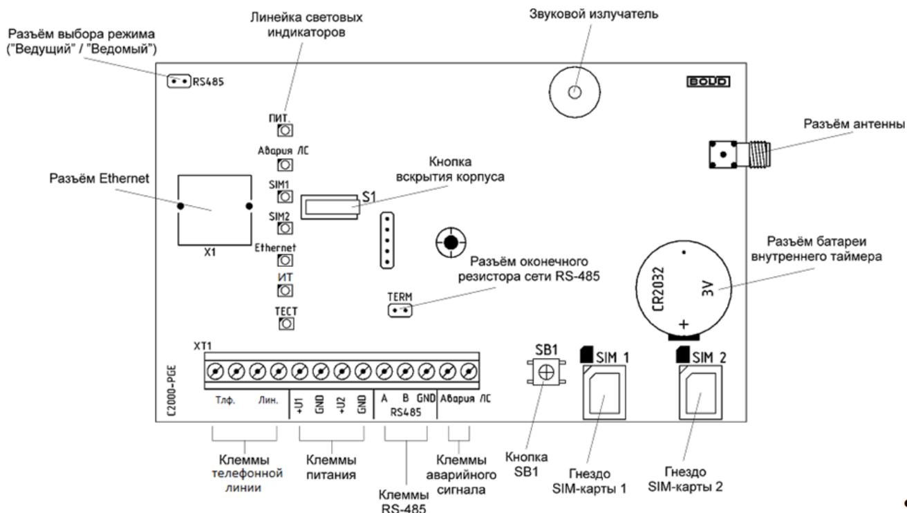
Рисунок 4-1 Схема платы «С2000-РGE»
