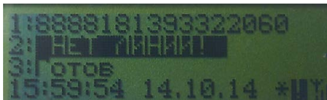
Рисунок 6. Отображение сообщения в формате Contact ID по телефонной линии
