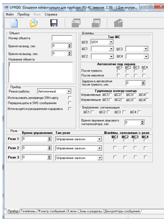
Рисунок 12. Uprog «YO-4C»
