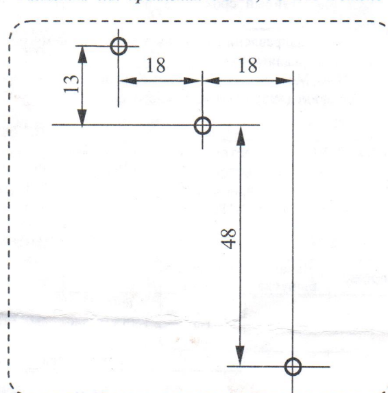
Разметка для крепления УО-1Р, УО-1/1Р к стене
