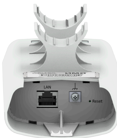
Разъемы нижней панели WB-2P-LR5
