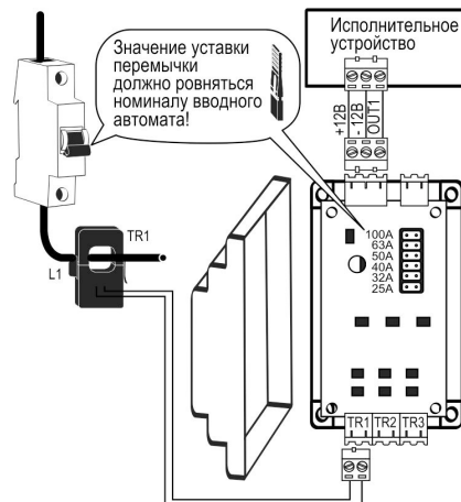
Рисунок 4 – Схема однофазного подключения
