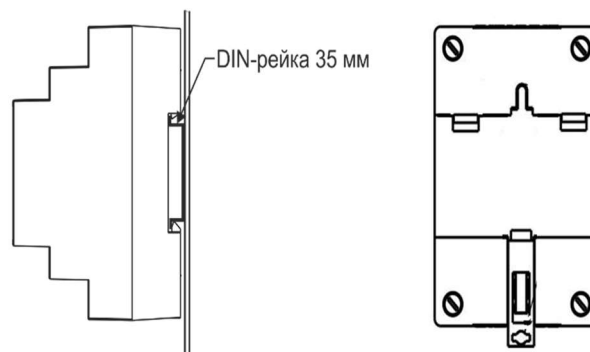
Рисунок 1 – Крепление изделия
