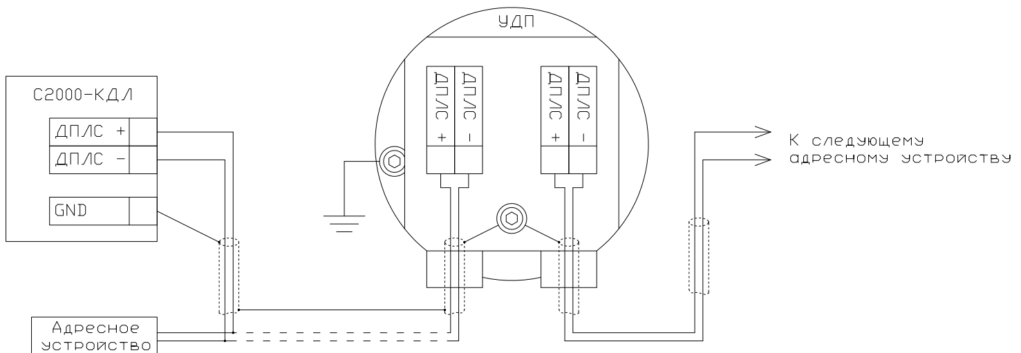
Рисунок 3 – Схема подключения УДП
