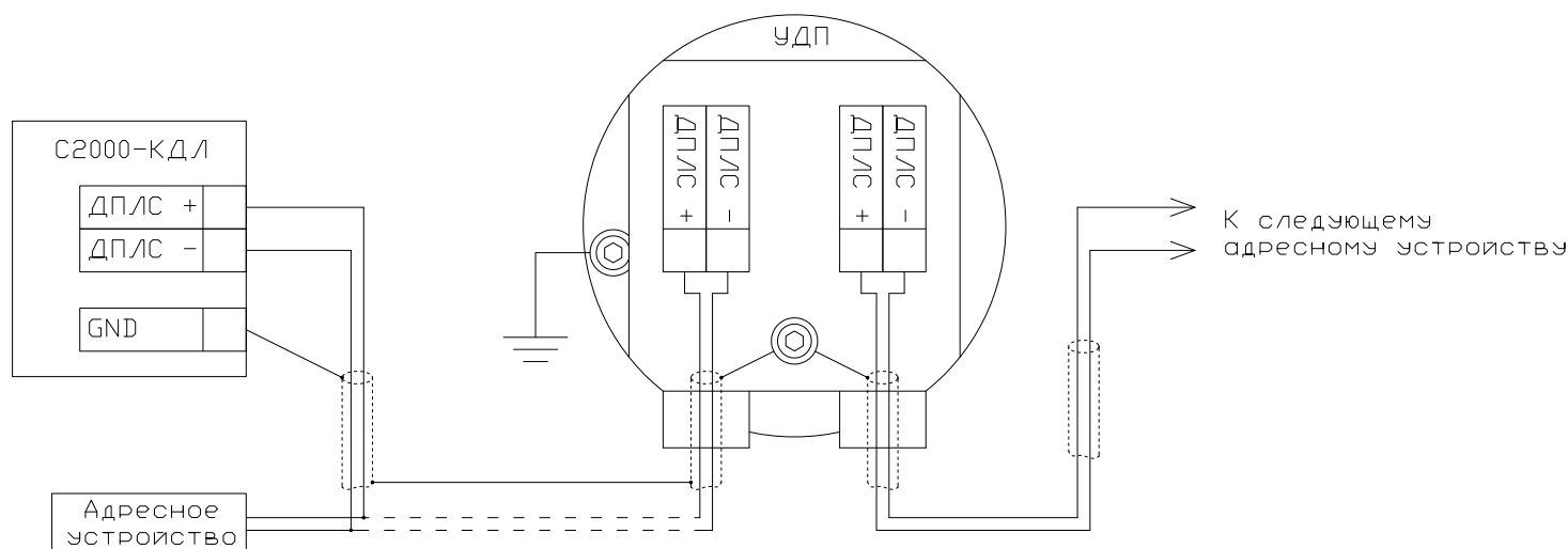
Рисунок 3 – Схема подключения УДП
