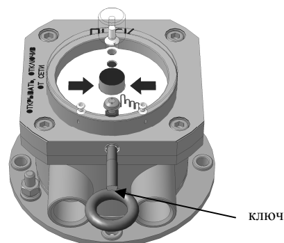
Рисунок 5 – Вид УДП со специальным инструментом (ключом)
