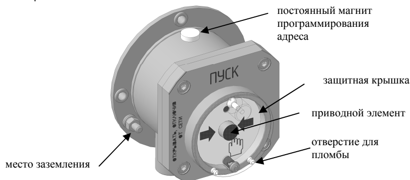
Рисунок 4 – Внешний вид УДП
