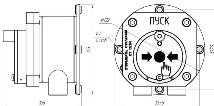
Рисунок 1 – Габаритные размеры УДП
