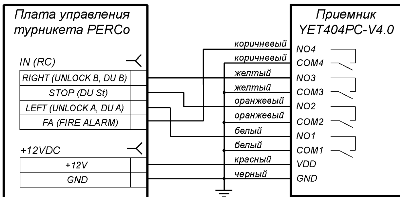
Рисунок 2. Рекомендованная схема подключения приемника YET404PC-V4.0 к плате управления ИУ
