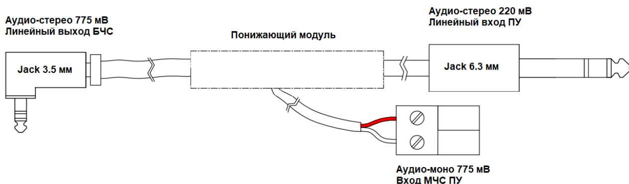
Рисунок 5 - Аудио кабель подключение (в комплекте)
