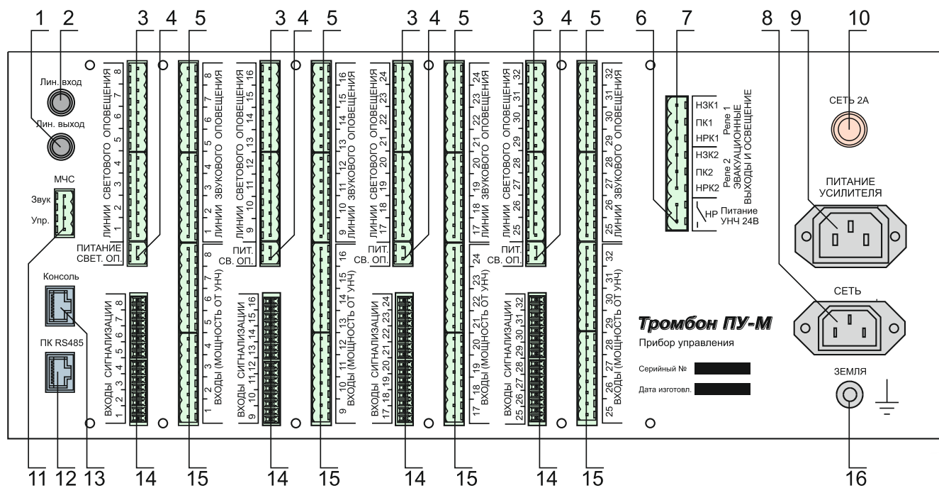
Рис. 2. Прибор управления «Тромбон ПУ-М», вид со стороны задней панели.
